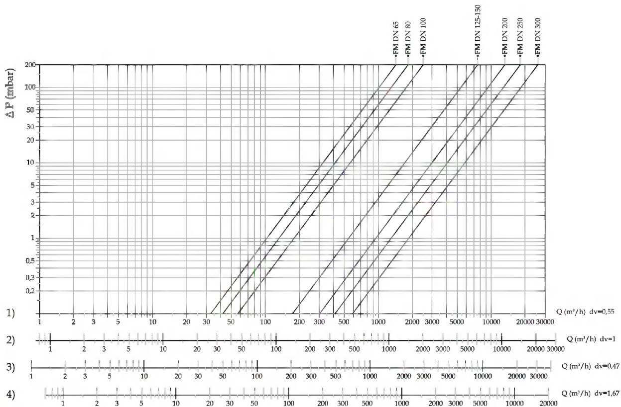
Діаграма перепаду тиску фільтрація 10 мкм (розрахована при P1 = 0 мбар)
