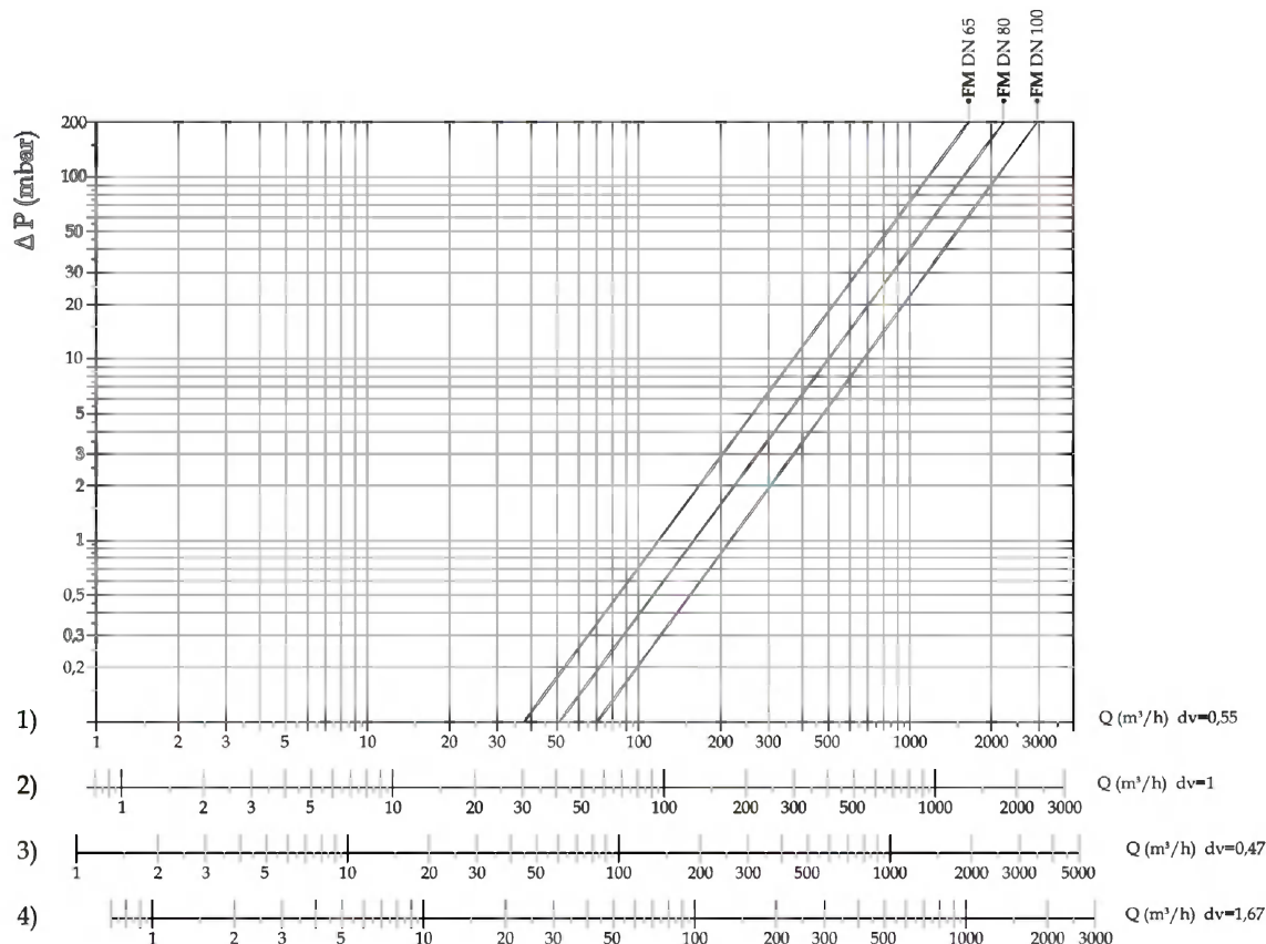
Діаграма перепаду тиску фільтрація 10 мкм (розрахована при P1 = 0 мбар)
