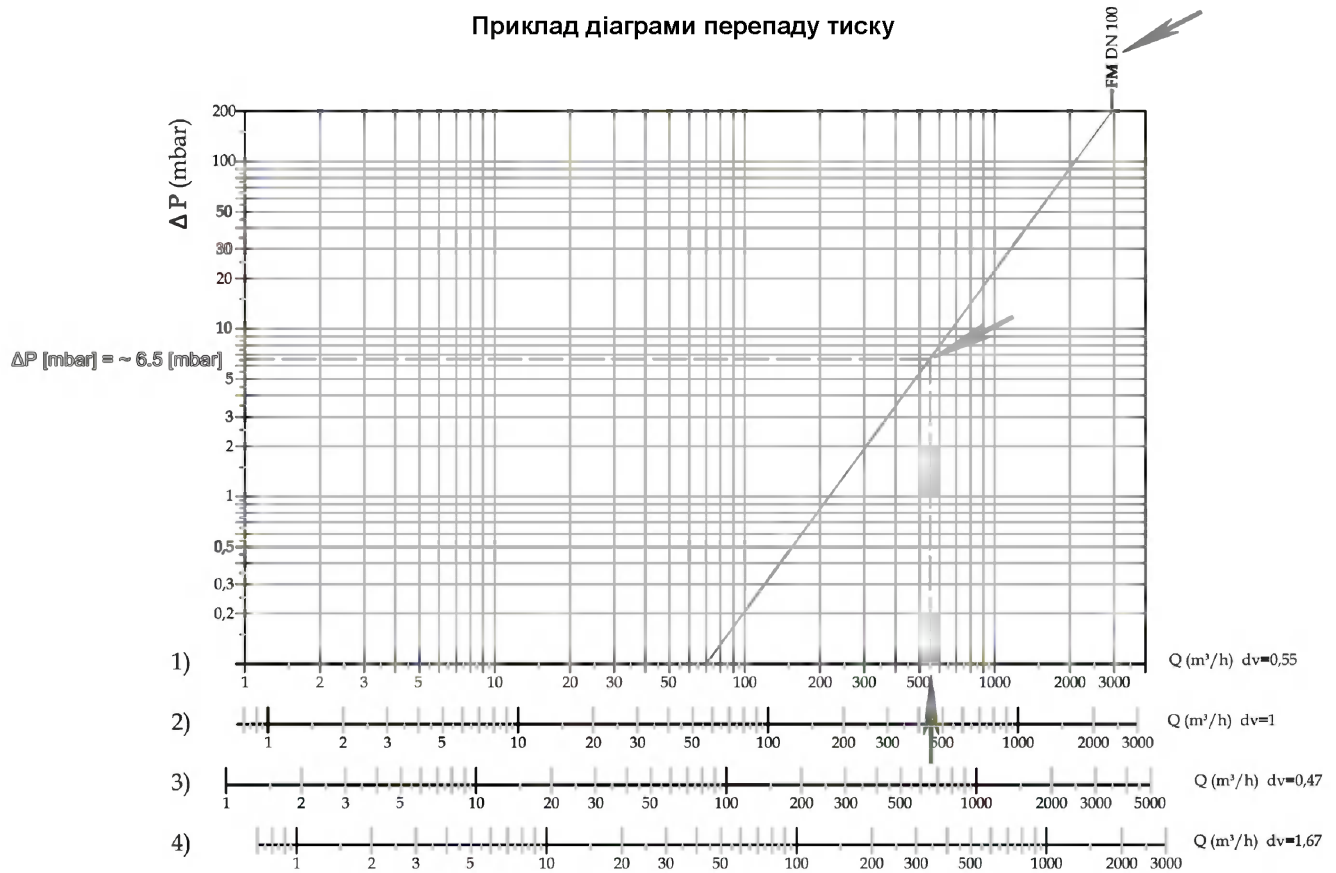
Діаграма перепаду тиску фільтрація 50 мкм (розрахована при P1 = 0 мбар)
